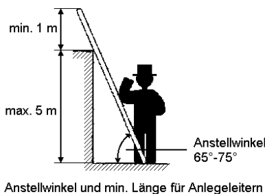
Anstellwinkel und min. Länge für Anlegeleitern
